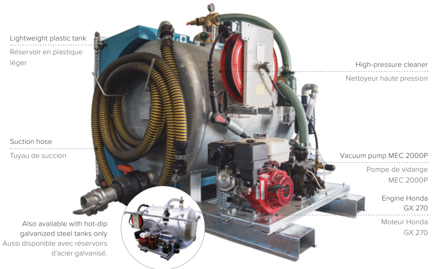
SIDE VIEW :: VUE LATÉRALE
